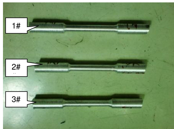
Tensile specimens
